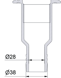
D-D ( 1 : 2 )
