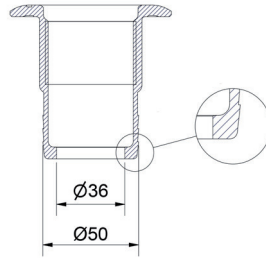
B-B ( 1 : 2 )
