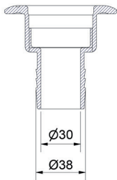
A-A ( 1 : 2 )
